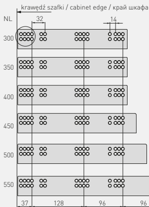
Rozstaw otworów montażowych Mounting dimensions Монтажные отверстия
