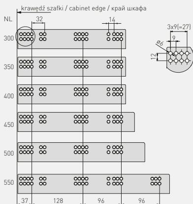
Rozstaw otworów montażowych Mounting dimensions Монтажные отверстия
