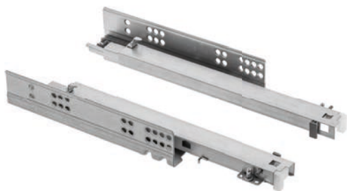
Kotek blokujący (zabezpieczenie przed wypadnięciem szuflady) Blocking peg (prevents drawer from falling out) Ограничитель (защита от выпадения ящика)
