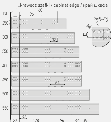
Rozstaw otworów montażowych Mounting dimensions Монтажные отверстия
